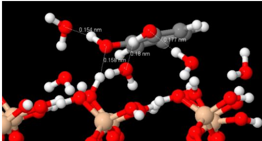
Waterstofbrug vorming tussen catechol en hydrofiele silica oppervlakte. 1
